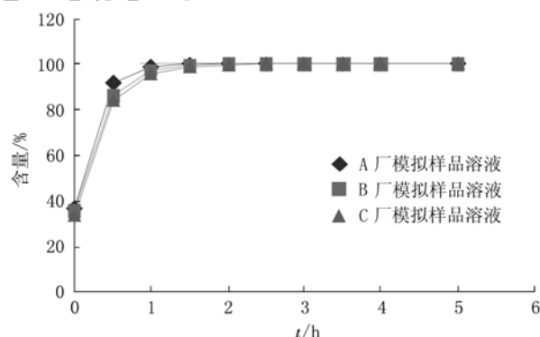
图 3 HPTC 闭环反应时间图
