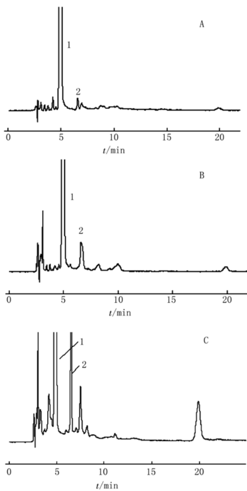
图 1 HPTC 注射液有关物质样品测定色谱图 A-批号 070301(A 厂); B-批号 20070116(B 厂); C-批号 20060820(C 厂); 1-HPTC; 2-喜树碱
