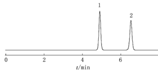
图 2 HPTC 注射液色谱图
